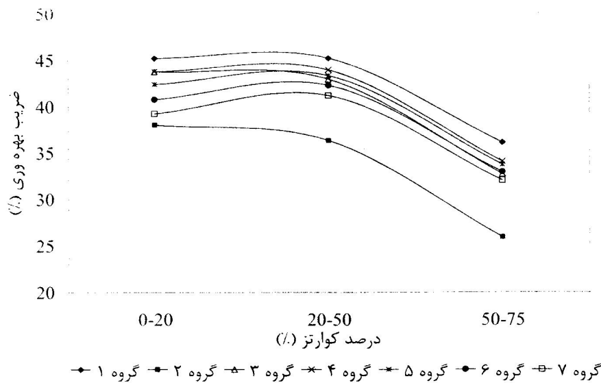
شکل ۲: ضریب بهره‌وری بر حسب درصد کوآرتز
