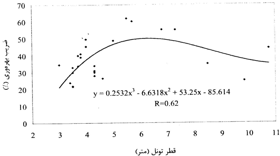
شکل ۱: ضریب بهره‌وری برحسب قطر تونل برای سنگ‌های با مقاومت فشاری ۱۲۰-۱۱۰ مگاپاسکال
